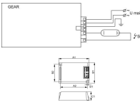
Caractéristiques Philips HID-PV C 35 /S CDM 50/60Hz Voir le produit
