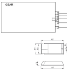
Technische Daten Philips HID-PV C 35 / I CDM 220-240V 50/60Hz für 35W Produkt ansehen
